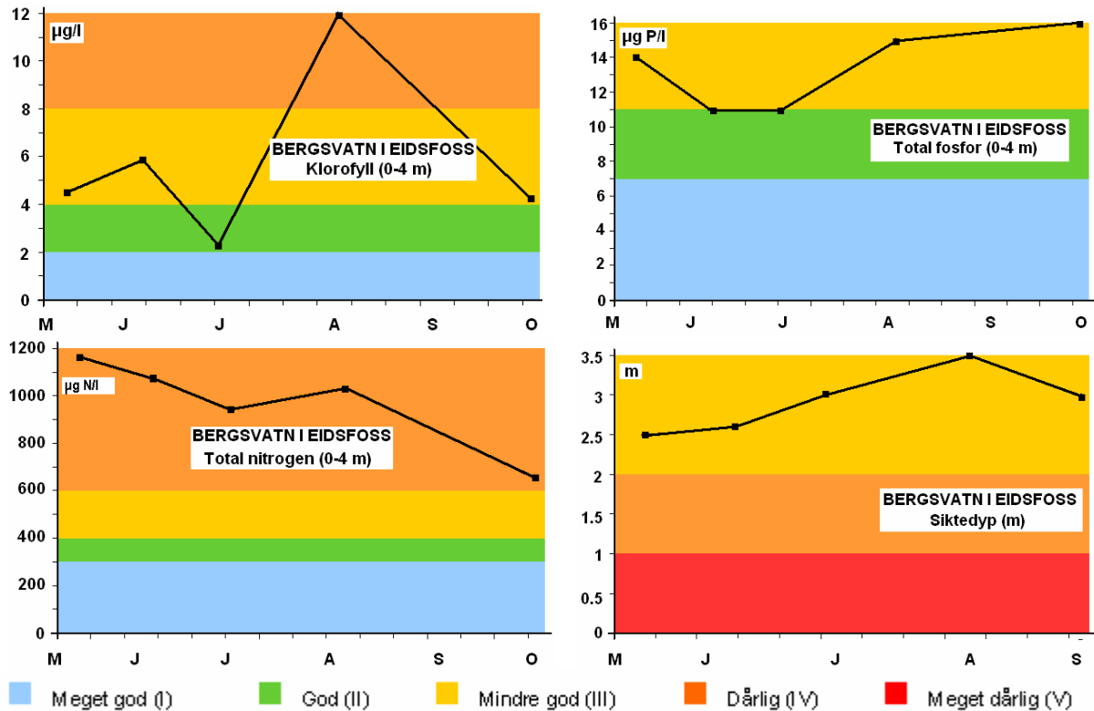
Figur 6. Bergsvatn i Eidsfoss 2005. Eutrofirelaterte parametre sammenliknet med SFTs vannkvalitetsparametre.
