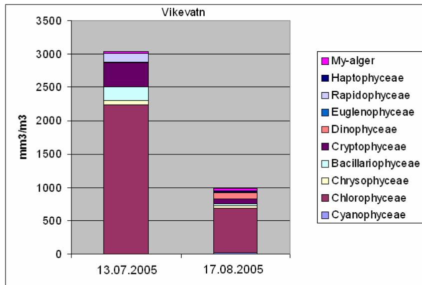
Figur 10. Vikevatn 2005. Planteplanktonets sammensetning (hovedgrupper) og biomasse (algevolum)
