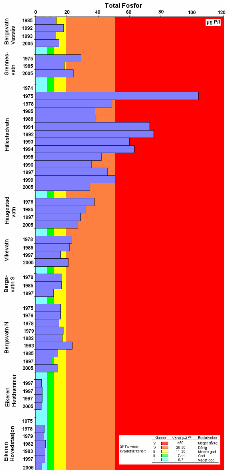
Figur 24. Middelerverdiar for Tot-P i de ulike innsjøene i de år innsjøene er undersøkt. Kraftig retensjon (selvrensing) av fosfor i innsjøene ned mot Eiker
