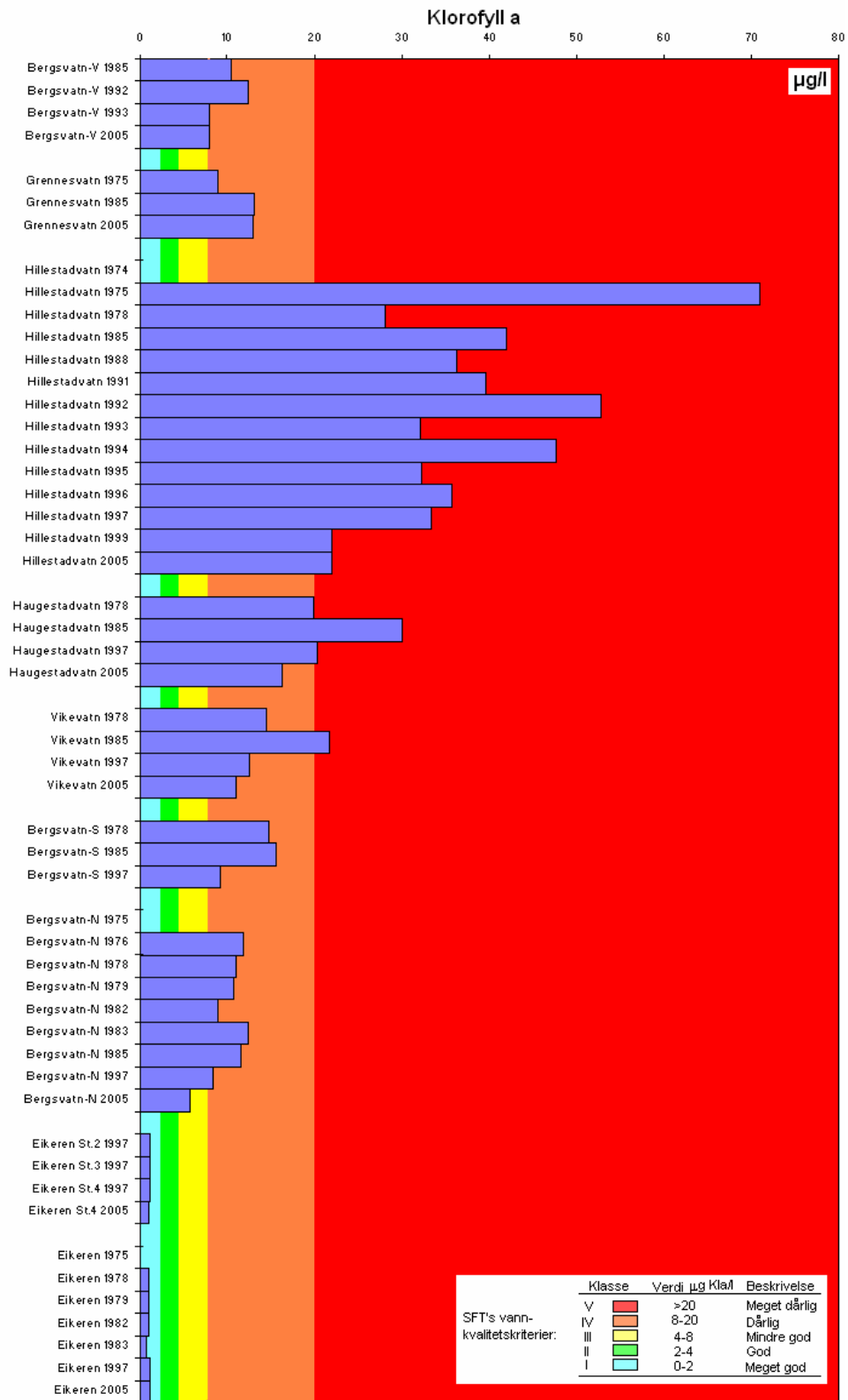
Figur 25. Middelveier for Klorofyll-a (algemengde) i de ulike innsjøene (alle undersøkelser).
